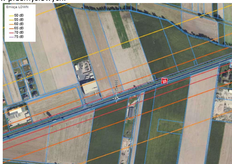
Rysunek 1 Analiza akustyczna drogi krajowej nr 25, źródło: geoportal.gov.pl
