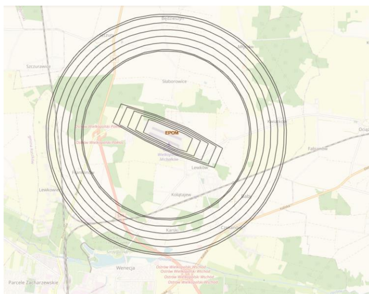
Rysunek 2 Powierzchnie ograniczające przeszkody, na podstawie mapy z www.ulc.gov.pl
