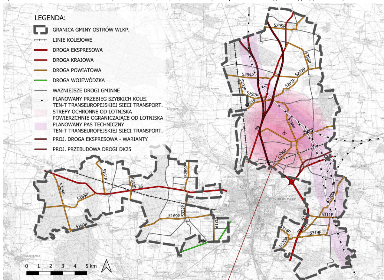
Ryc. 14. Rozmieszczenie infrastruktury transportowej w tym planowanej oraz powierzchnie ograniczającej przeszkody od lotniska
