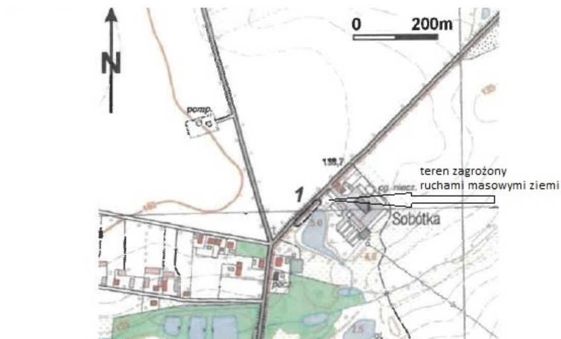
Ryc. 5. Teren zagrożony ruchami masowymi ziemi.
